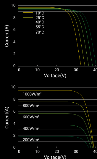
I-V Curve: (A-M380)
